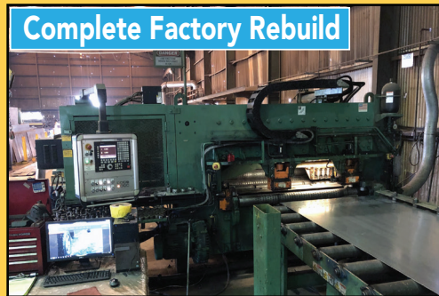
Peddinghaus FPB 1500
