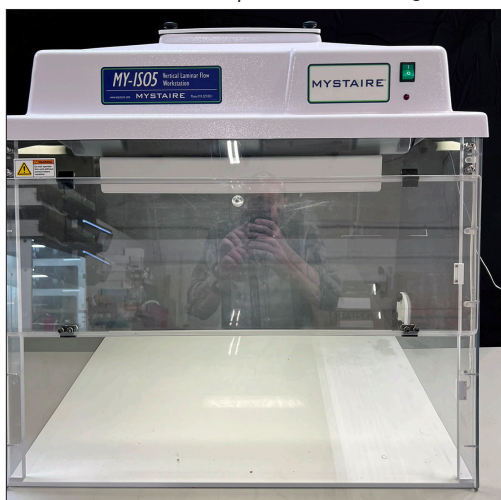
MyStaire PCR Hood, Mdl. MY-1S05
